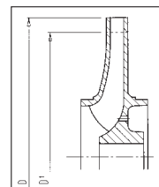
Reducción con torneado del diámetro exterior del rodete para bomba centrifuga.
