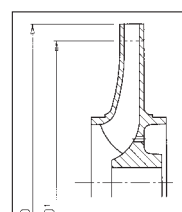
Уменьшение внешнего диаметра колеса подрезкой
